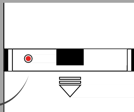
Painel Traseiro da Fechadura
