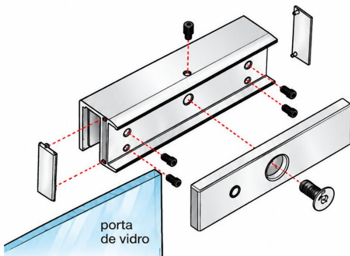
Instalação do suporte em U
