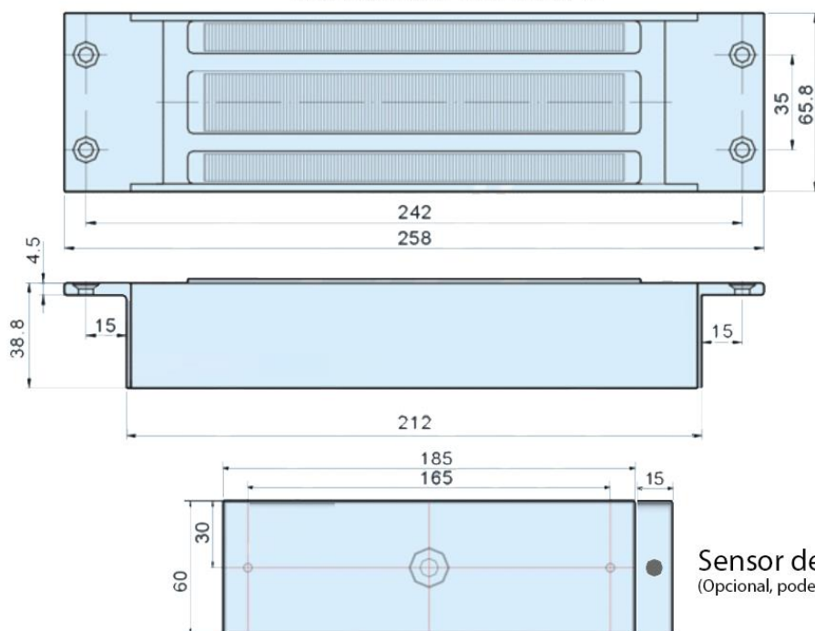
Placa fixação
