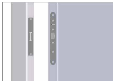
Instalação lateral
