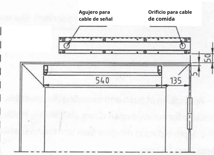
Puerta que se abre hacia la derecha
