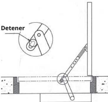
Puerta que se abre hacia la derecha
