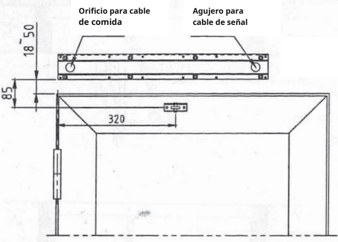
Puerta que se abre hacia la izquierda
