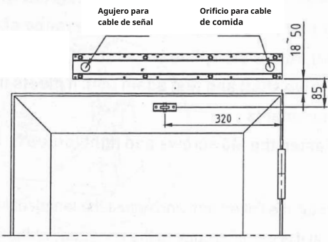
Puerta que se abre hacia la derecha
