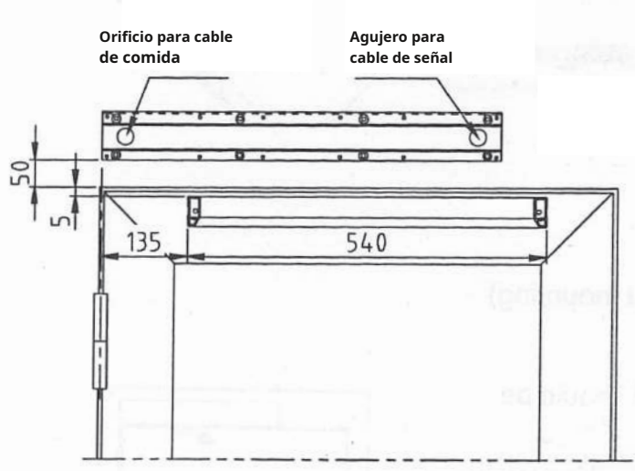
Puerta que se abre hacia la izquierda
