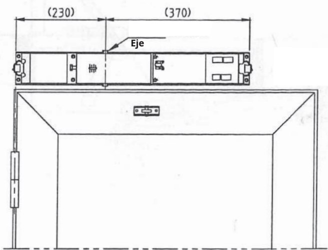
Puerta que se abre hacia la izquierda
