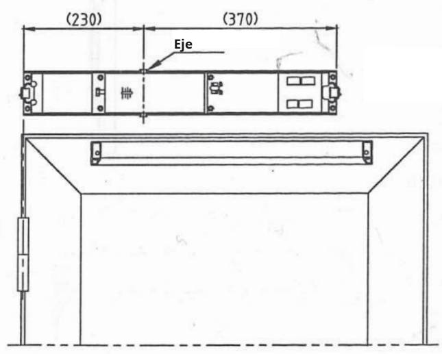
Puerta que se abre hacia la izquierda
